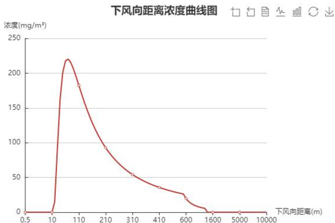
图 4.2.6-4 最常见气象条件下甲醛泄漏 10min 下风向距离浓度曲线图
