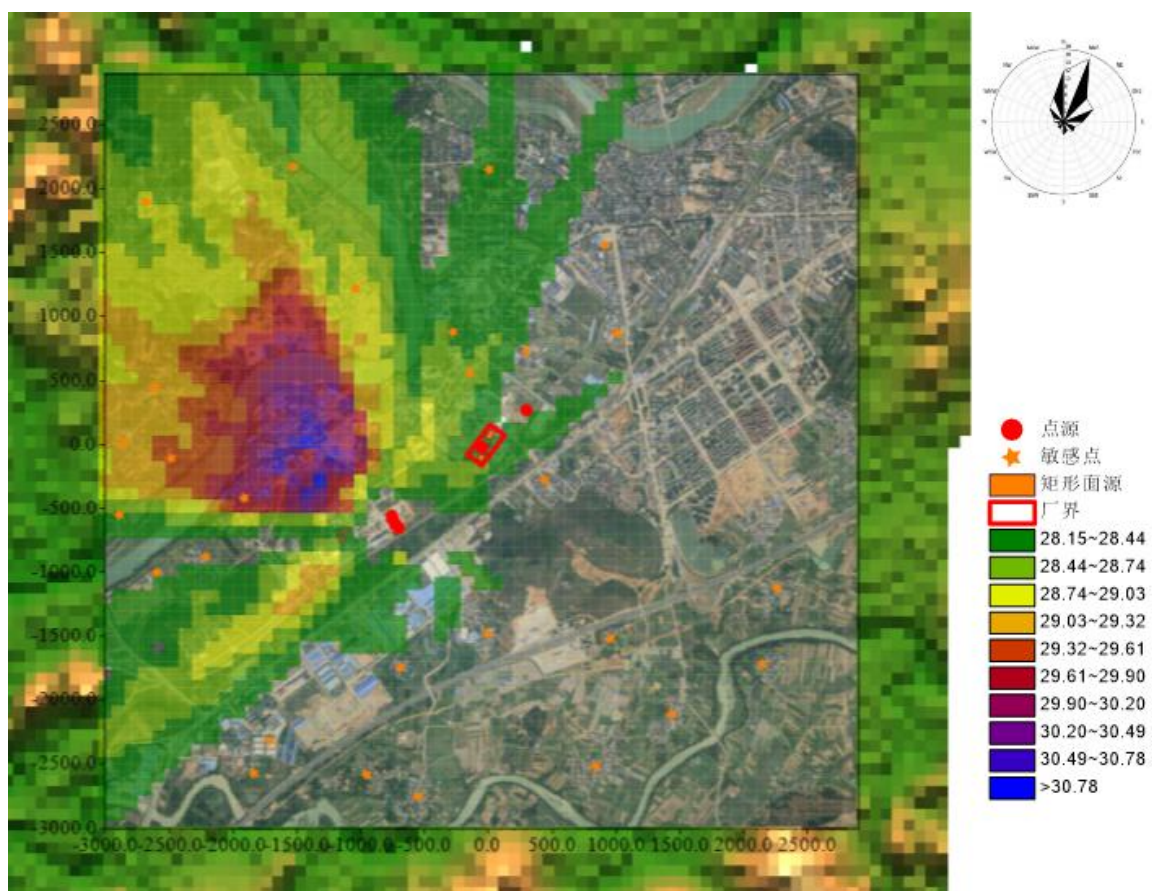
图 4.2.1-25 正常排放条件下 \text{NO}_2 (98%保证率日平均, 叠加预测值) 浓度等直线图
