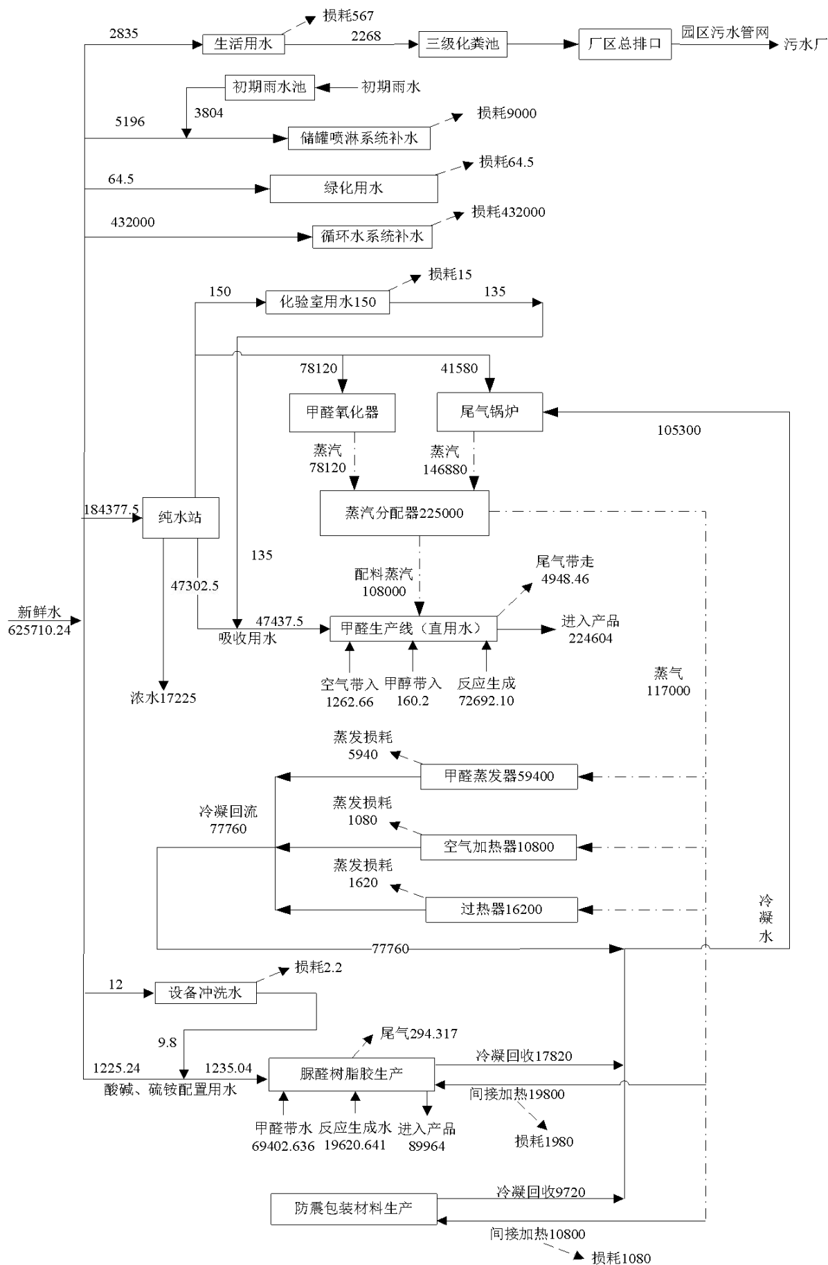
图 2.5.1-2 扩建完成后全厂水平衡 单位: m 3 /a
