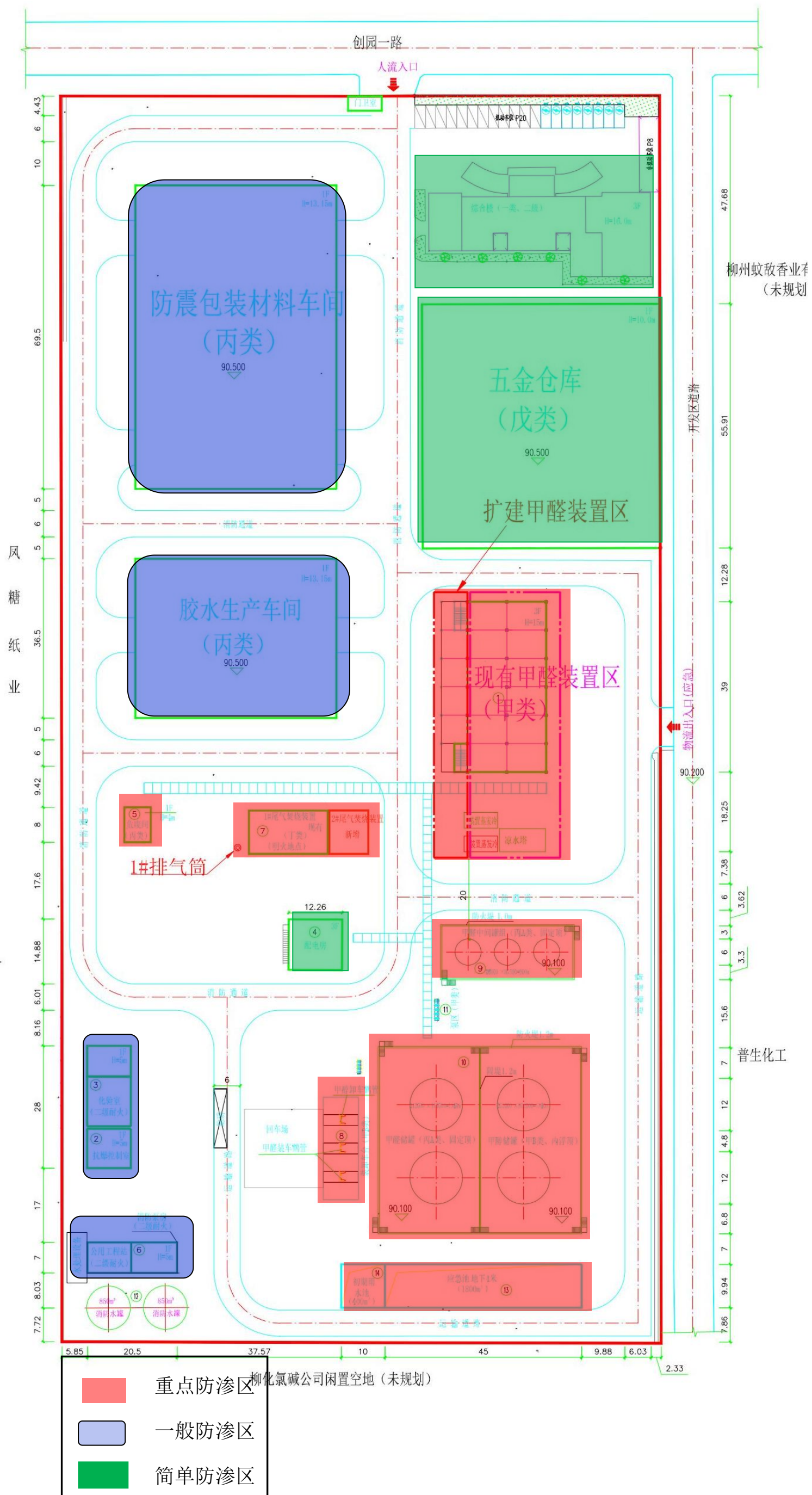
附图 16 项目分区防渗图
