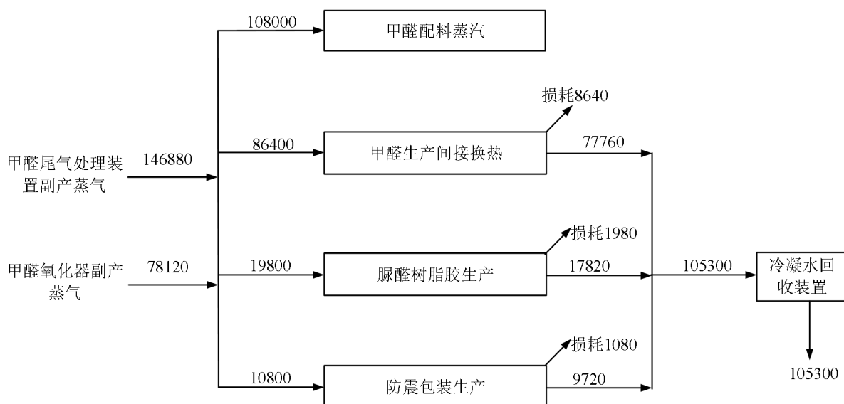
2.2.8-2 扩建后全厂蒸汽平衡（单位：t/a）
