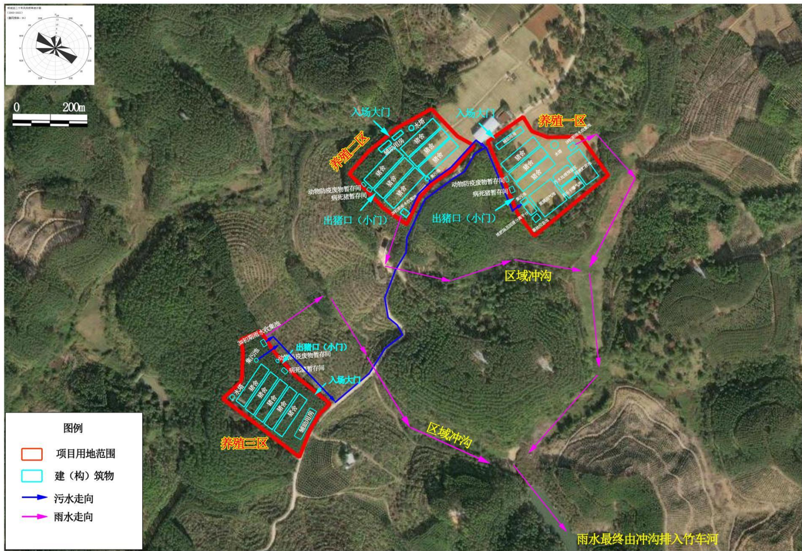
附图3 项目总平面布置及雨污水走向图
