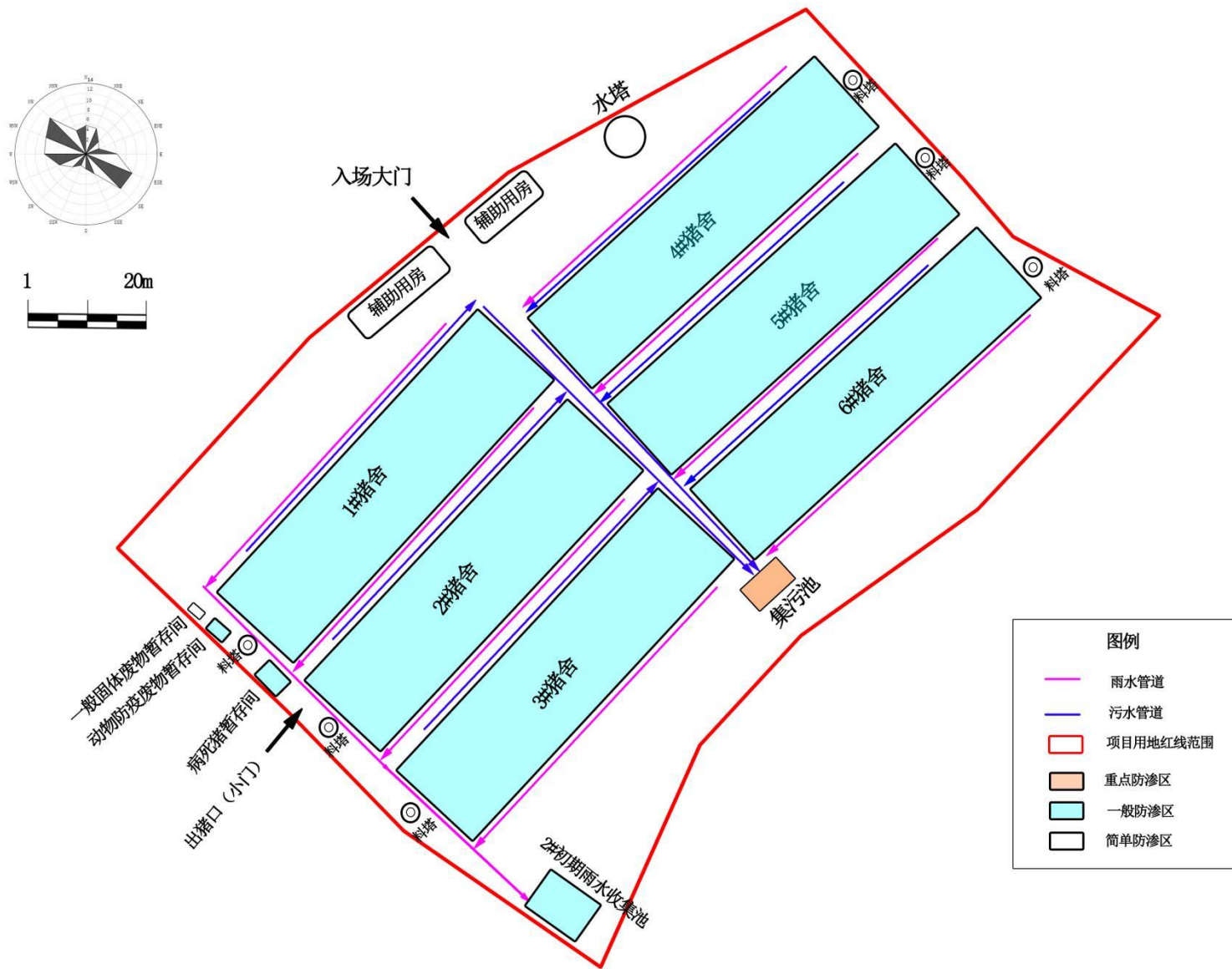
附图2-2 项目养殖二区总平面布置及分区防渗图
