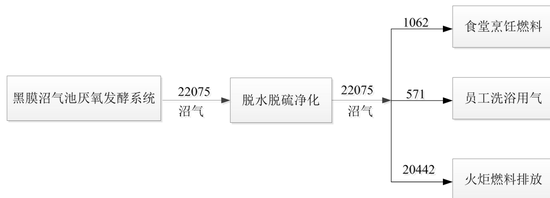
图 2.2-14 项目沼气平衡图（单位：m 3 /a）
