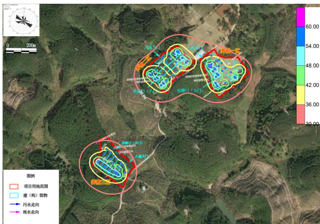
图 4.2-2 项目噪声等值线图
