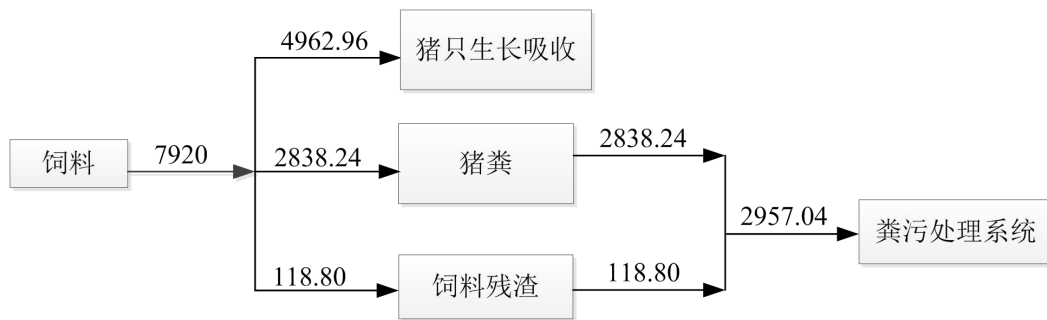
图 2.2-13 项目全场物料（饲料）平衡图（单位：t/a）
