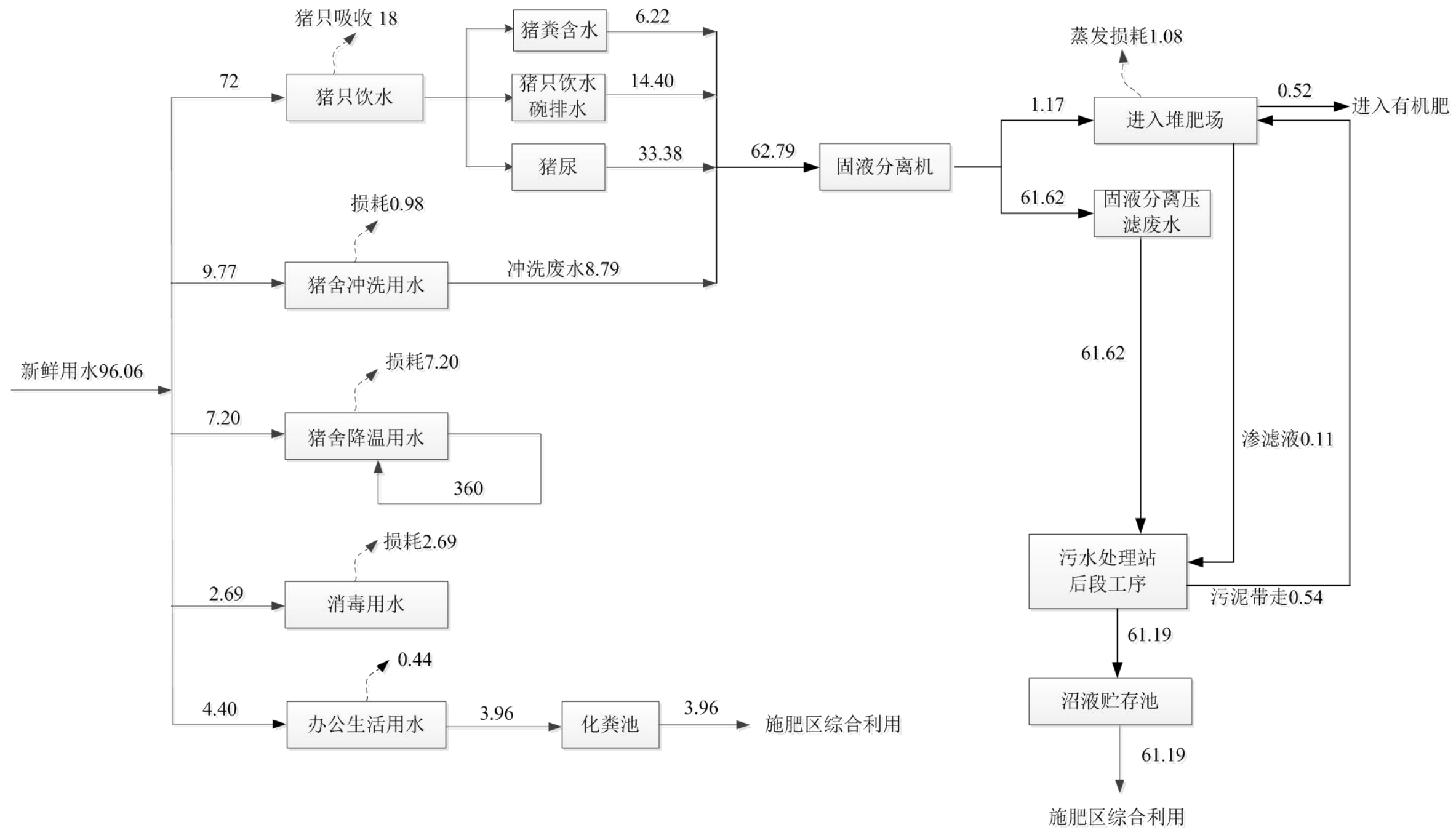
图2.2-17 项目全场其它季节水平衡图（单位：m 3 /d）
