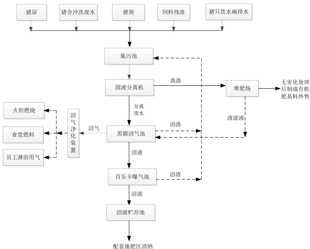
图2.2-8 项目污水处理工艺流程及产污环节图
