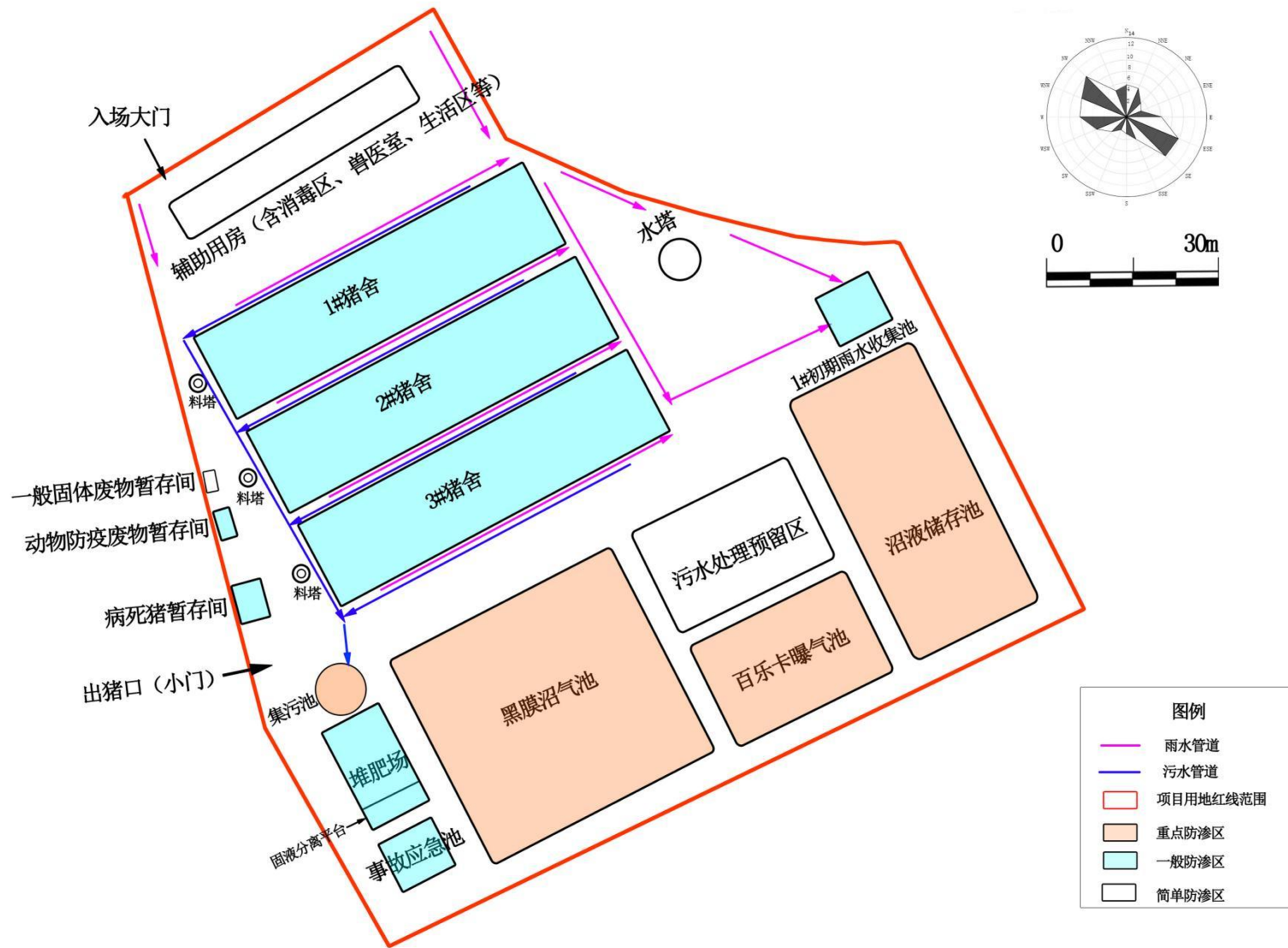
附图2-1 项目养殖一区总平面布置及分区防渗图
