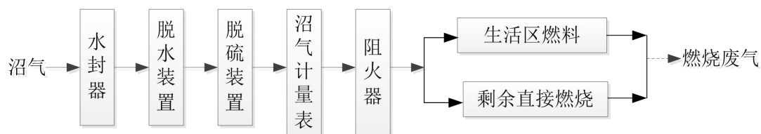
图 2.2-12 沼气利用流程及产污环节图
