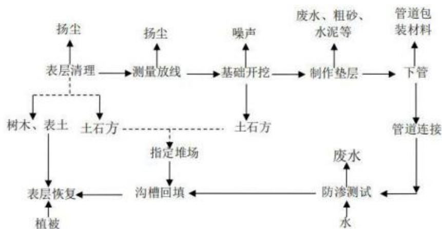
图 2.2-2 管线施工流程及排污节点图
