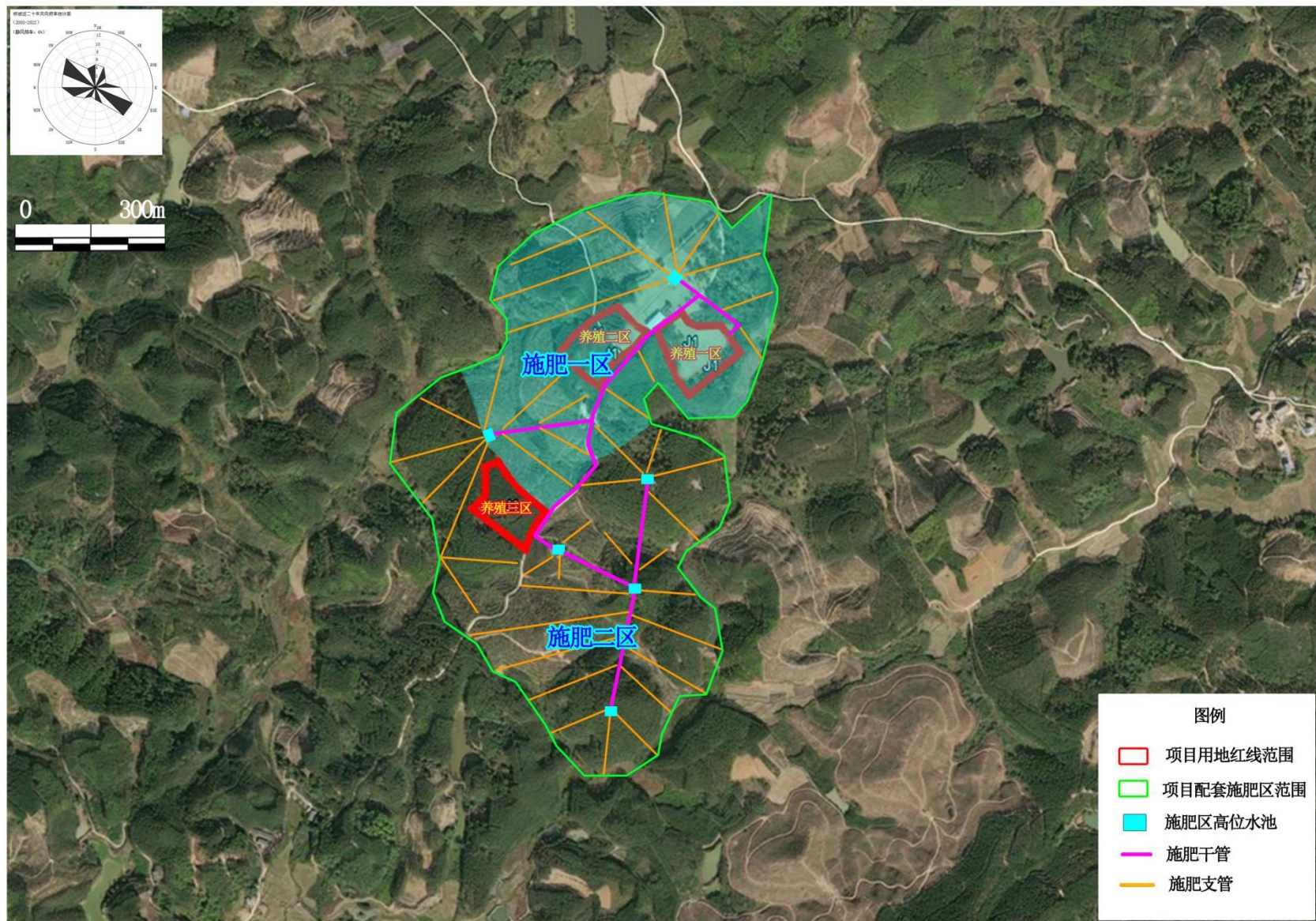
附图10 项目施肥区位置及施肥管网分布图
