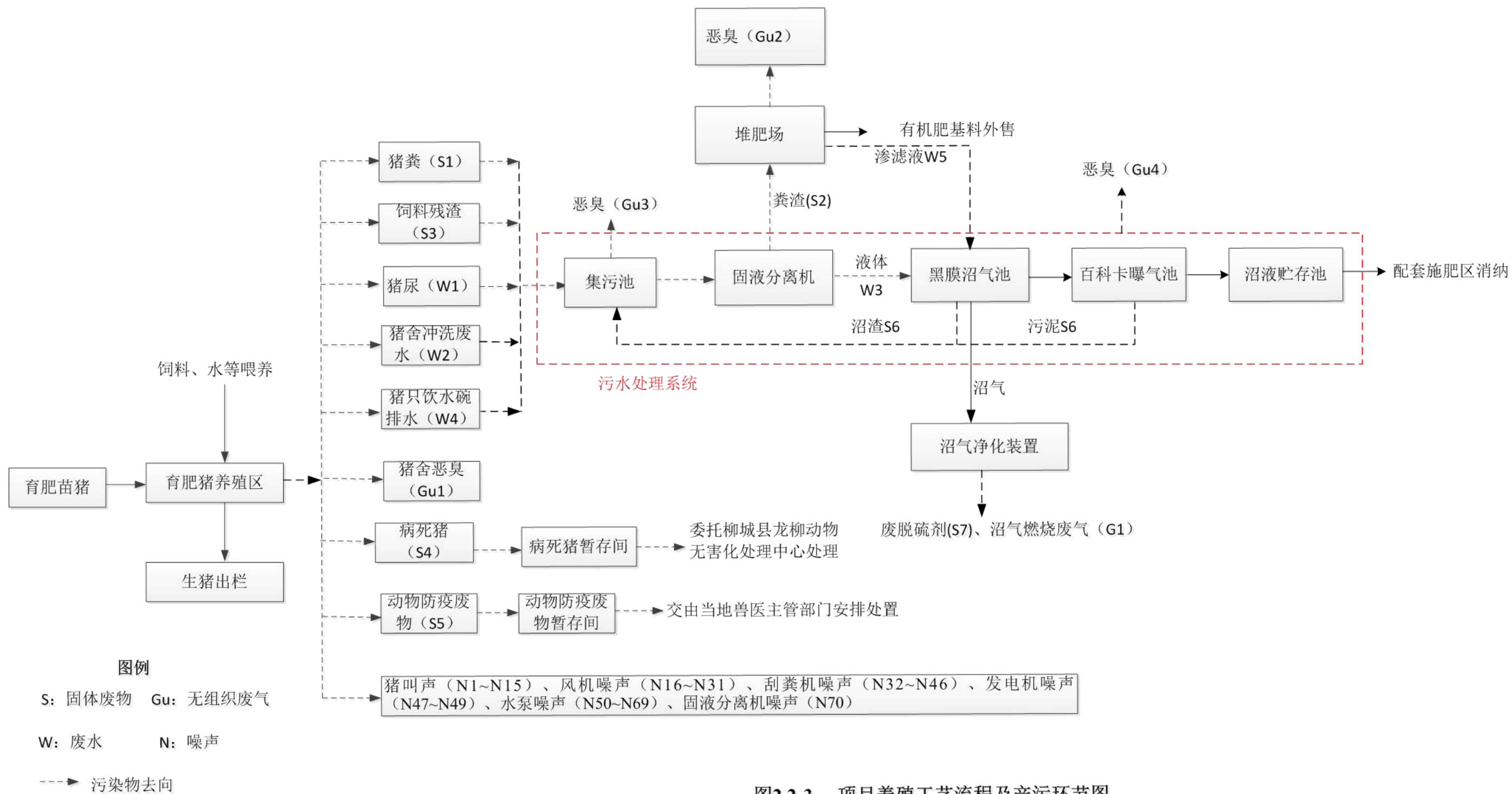
图2.2-3 项目养殖工艺流程及产污环节图
