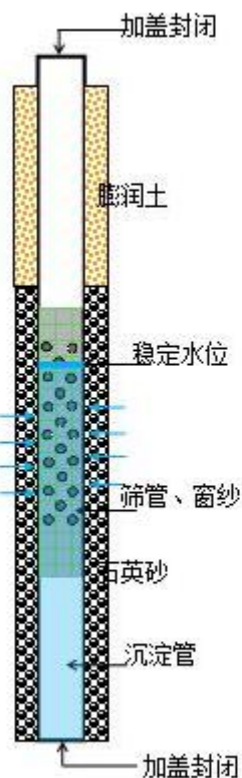
图 5.2-1 地下水监测井结构图
